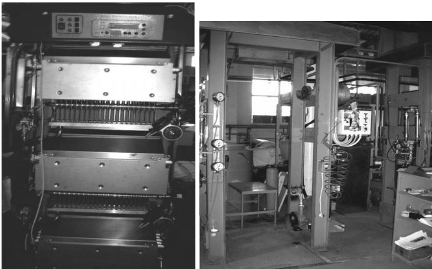
Рис. 4. Модуль нагріву МН ( a ) та лабораторний стенд для його випробування ( б )
