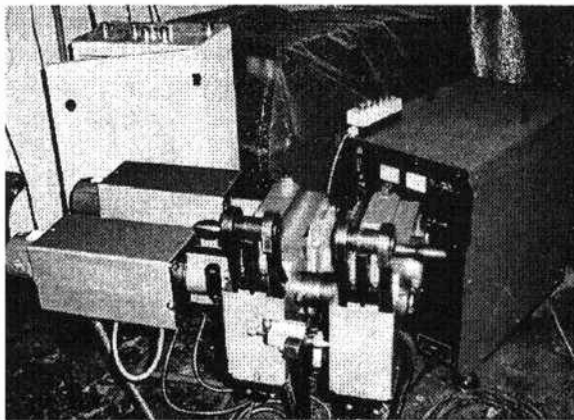
Рис. 3. Установа для зварювання труб МДВ 1
