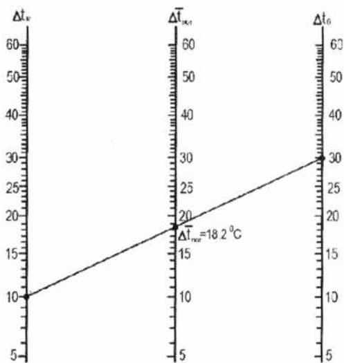
Рис. 3. Номограма функції \Delta \bar{t}_{\text{нов}} = \frac{\Delta t_{\delta} - \Delta t_m}{\ln \frac{\Delta t_{\delta}}{\Delta t_m}}
